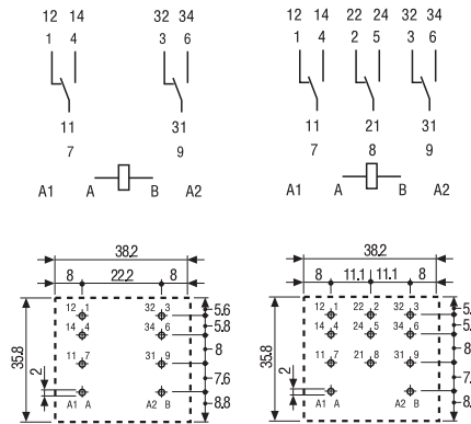
62.22 Ansicht auf die Anschlüsse 62.23 Ansicht auf die Anschlüsse 62.22 - 0300 Ansicht auf die Anschlüsse 62.23 - 0300 Ansicht auf die Anschlüsse
